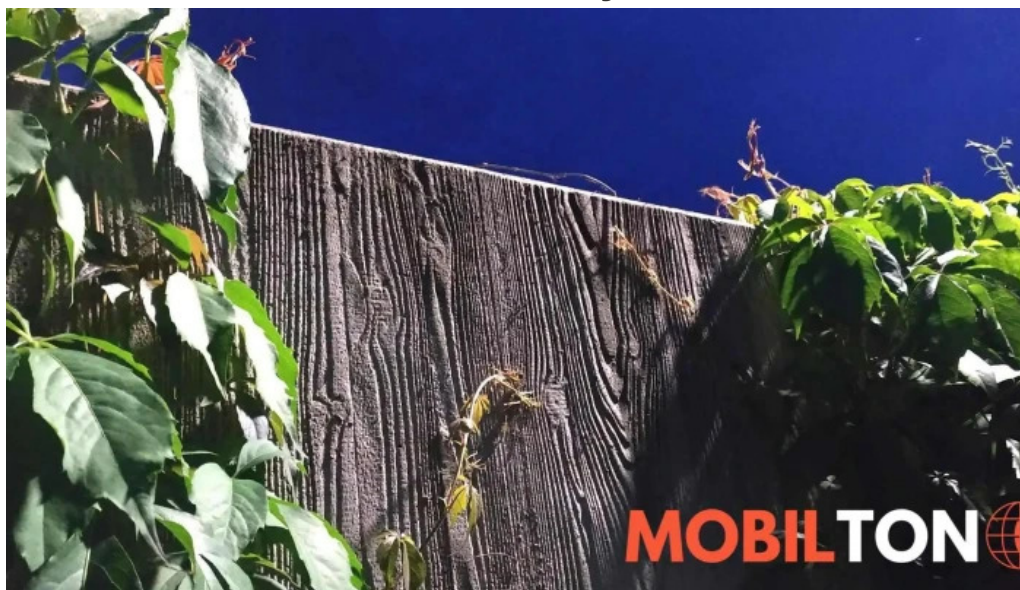
Pallasit vse
